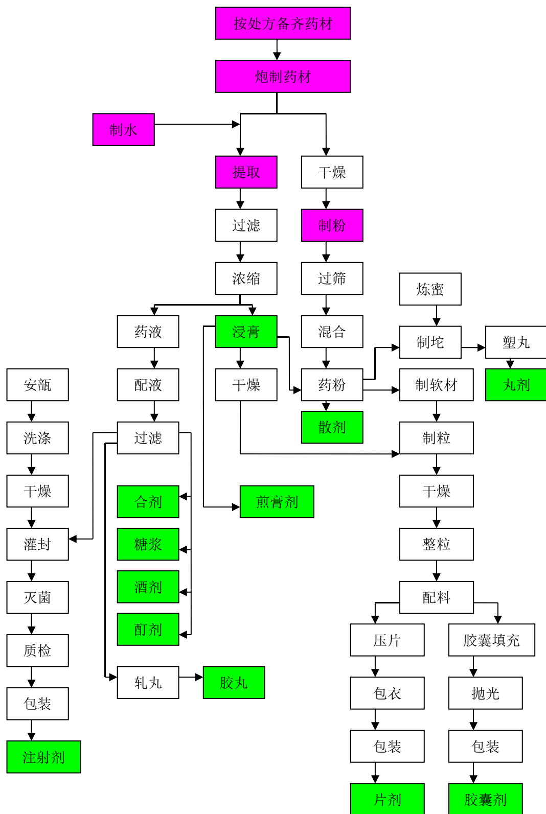
图 1-1 常见剂型制备工艺流程简图
